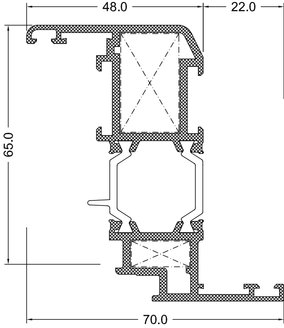
HEMYÜZ KANAT PROFİLİ
