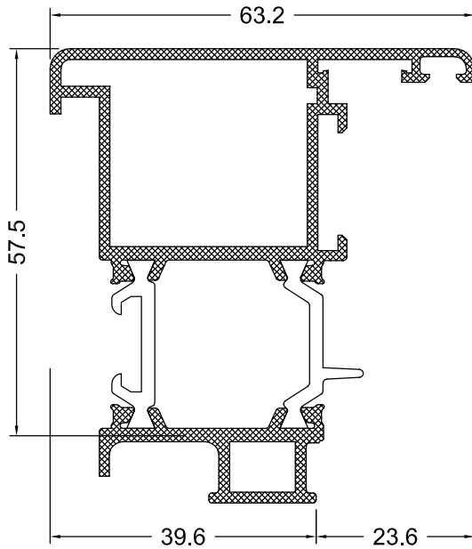
PİVOT AÇILIM ADAPTÖRÜ
