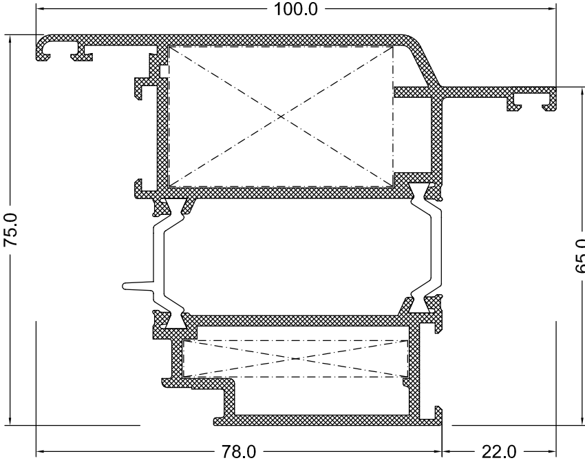
HEMYÜZ DIŞA AÇILIR KAPI KANAT PROFİLİ
