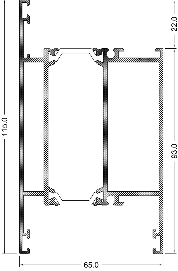
DAR ETEK PROFİLİ
