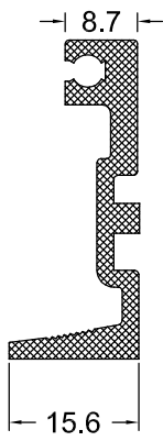
SW ZIVANA PROFİLİ
