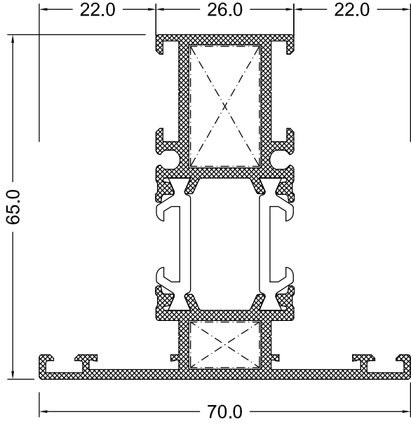
ORTA KAYIT PROFİLİ
