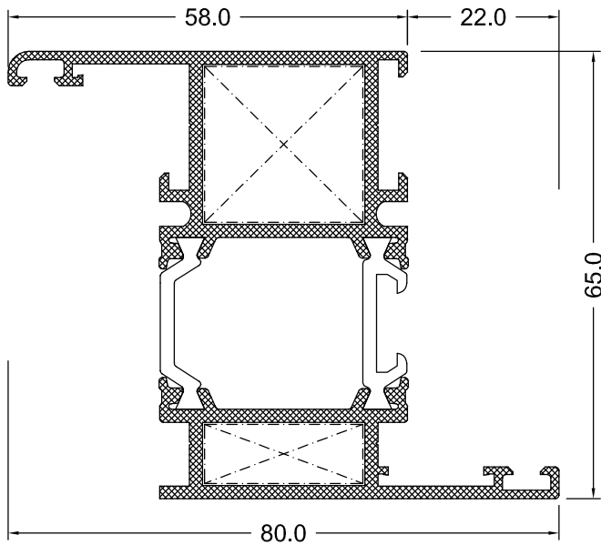
Z KASA PROFİLİ
