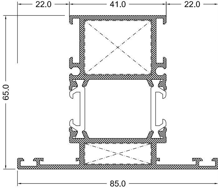
ORTA KAYIT PROFİLİ
