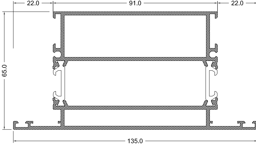
ORTA KAYIT PROFİLİ
