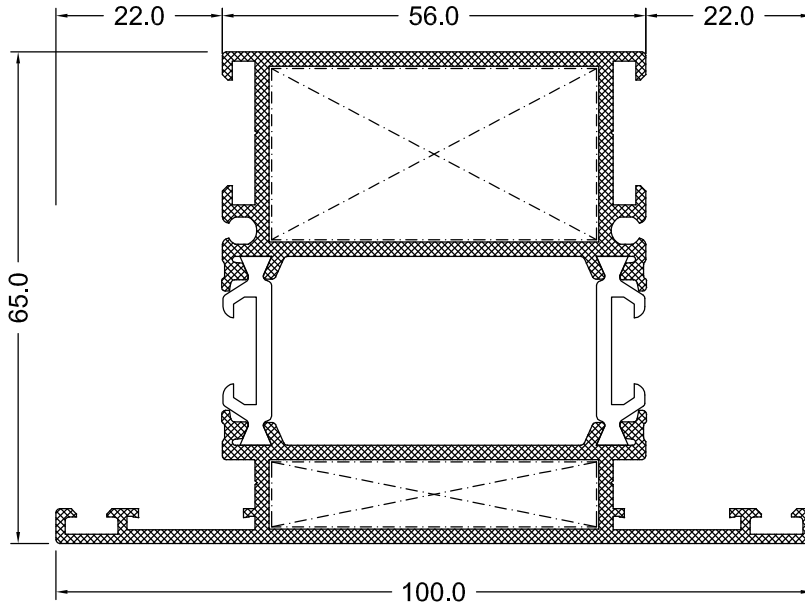
ORTA KAYIT PROFİLİ
