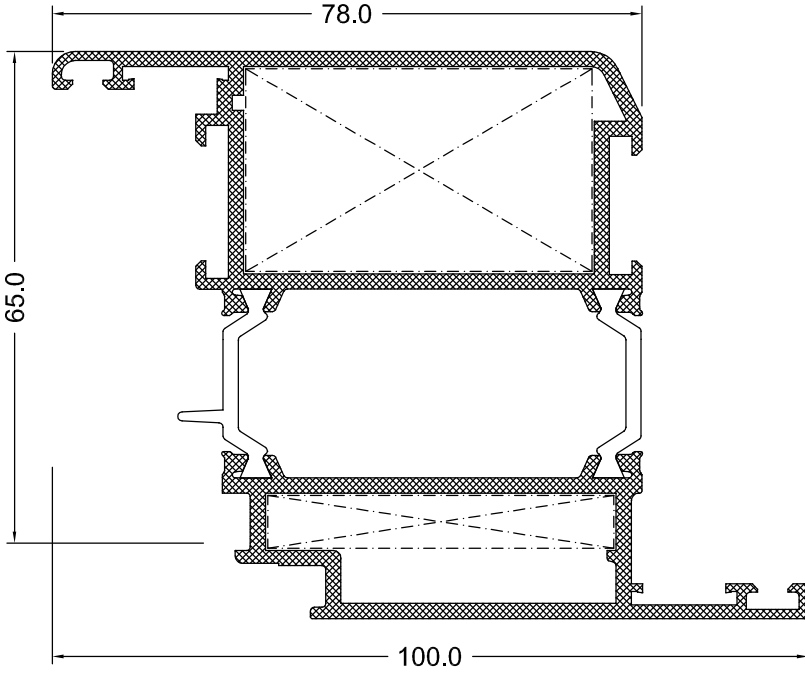
HEMYÜZ KAPI KANAT PROFİLİ
