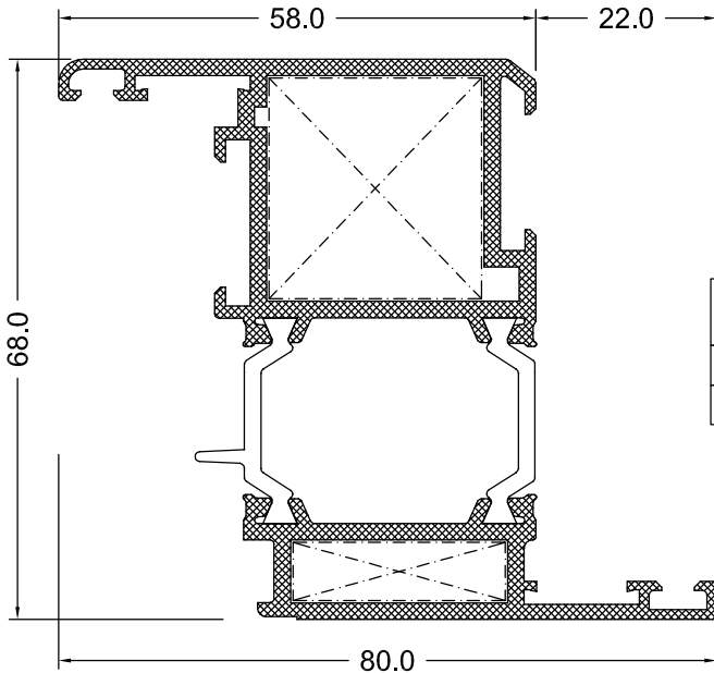
KANAT PROFİLİ
