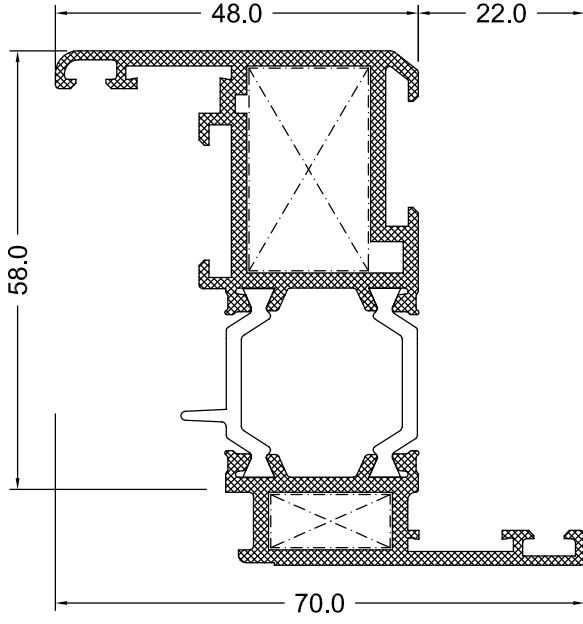
KANAT PROFİLİ
