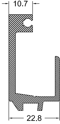
SW ZIVANA PROFİLİ
