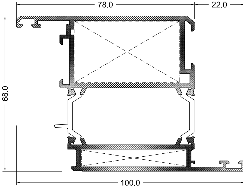
KAPI KANAT PROFİLİ
