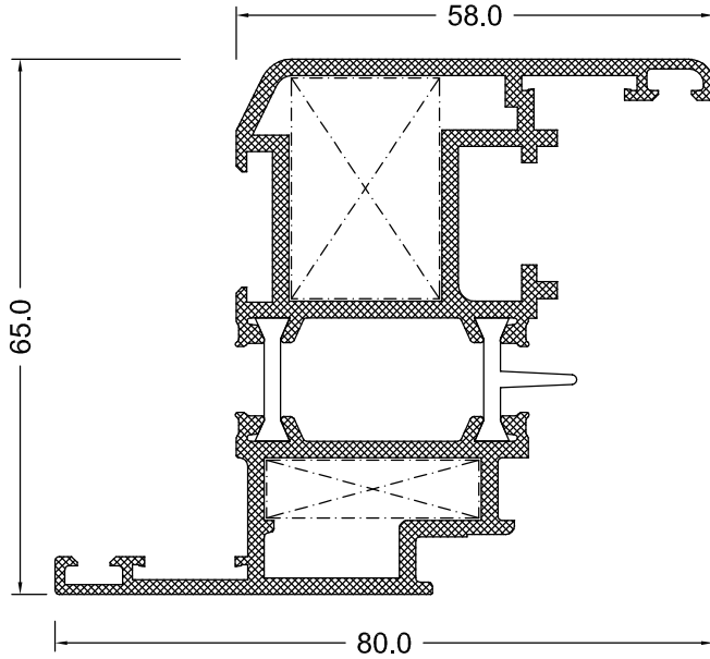
HEMİYÜZ KANAT PROFİLİ
