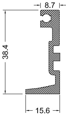
SW ZIVANA PROFİLİ ALT
