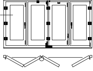
AY-55 YALITIMLI DOĞRAMA SİSTEMİ İLE KATLANIR KAPI DETAYI
