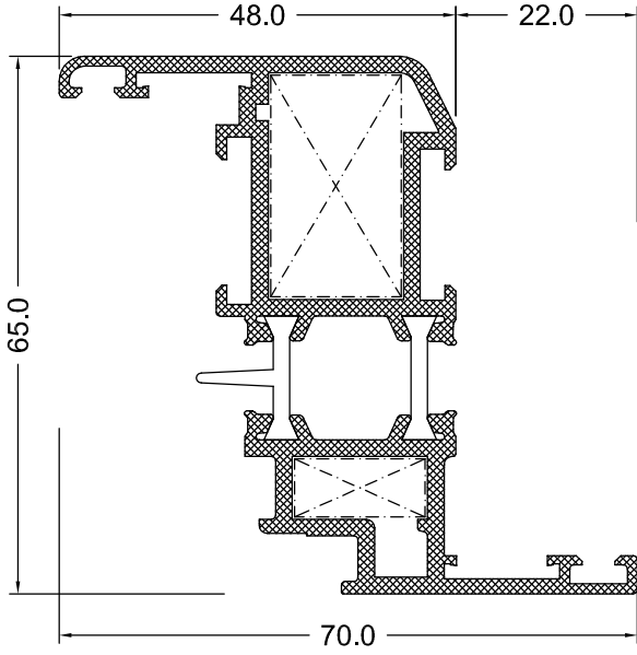
HEMİYÜZ KANAT PROFİLİ
