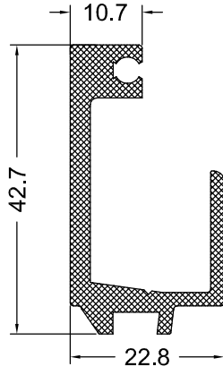
SW ZIVANA PROFİLİ ÜST
