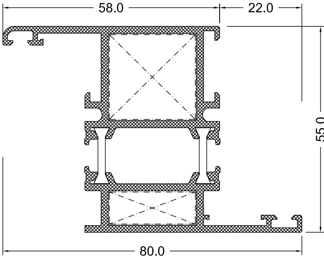
Z KASA PROFİLİ
