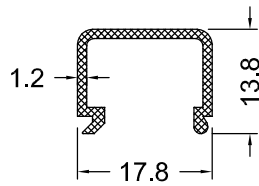
DS 82-15 0.152 Kg/m
