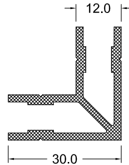
DS 91-12 0.602 Kg/m
