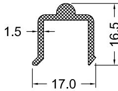
DS 81-15 0.187 Kg/m
