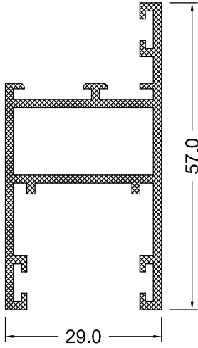
DS 31-15 0.748 Kg/m
