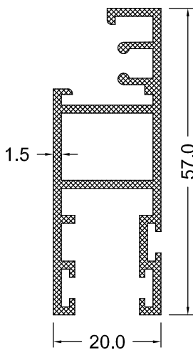
DS 81-00 0.726 Kg/m
