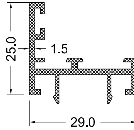
DS 65-15 0.363 Kg/m
