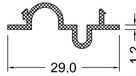
DS 66-12 0.168 Kg/m
