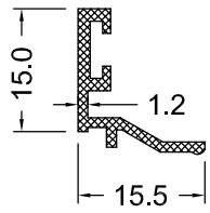
DS 40-12 0.144 Kg/m
