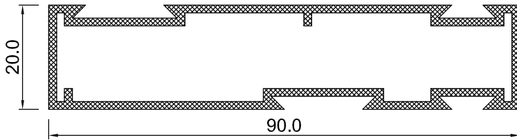
DS 23-15 1.041 Kg/m
