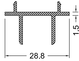
DS 56-15 0.249 Kg/m
