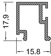
DS 41-15 0.211 Kg/m
