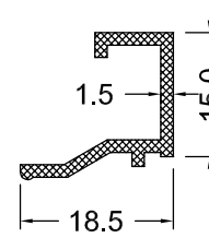
DS 48-15 0.179 Kg/m
