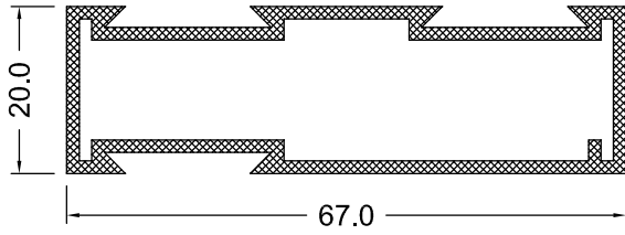
DS 21-15 0.805 Kg/m
