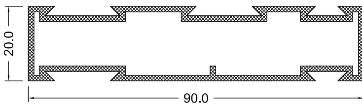
DS 22-15 1.068 Kg/m
