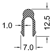
DS 80-00 0.089 Kg/m
