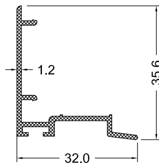
DS 55-12 0.279 Kg/m
