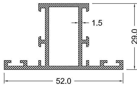
DS 01-15 0.637 Kg/m
