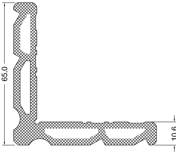
MS-503 2,195Kg/m
