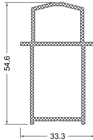
MS-505 0,730 Kg/m
