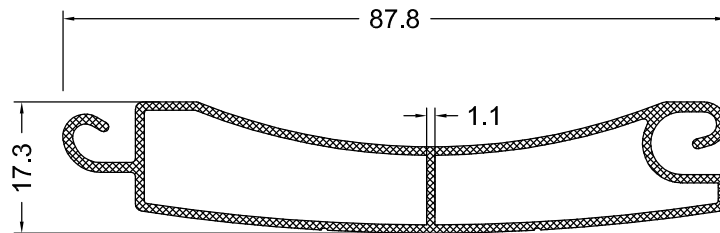
9305-11 0.686 Kg/m
