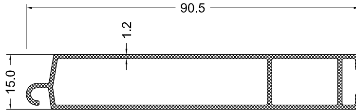
9302-12 0.718 Kg/m
