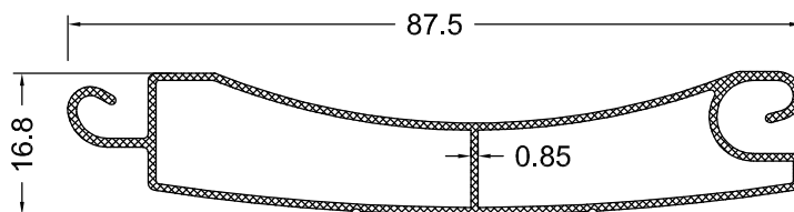
9305-085 0.535 Kg/m
