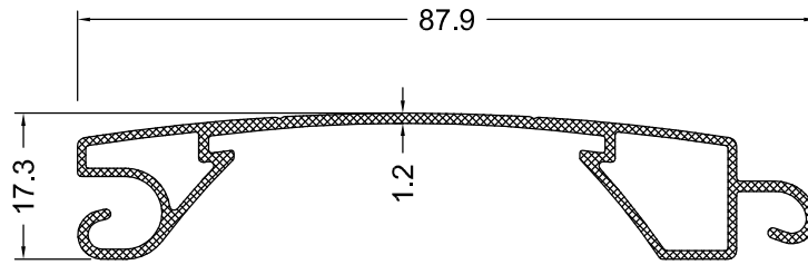
9306-13 0.583 Kg/m
