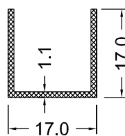
9314 0.143 Kg/m
