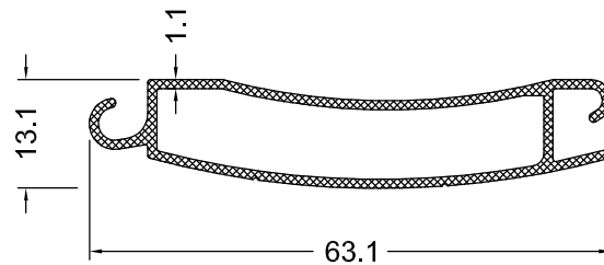
9310-11 0.437 Kg/m
