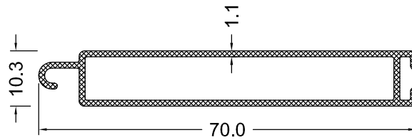
9313-11 0.464 Kg/m
