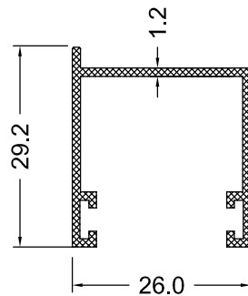
9312 0.294 Kg/m
