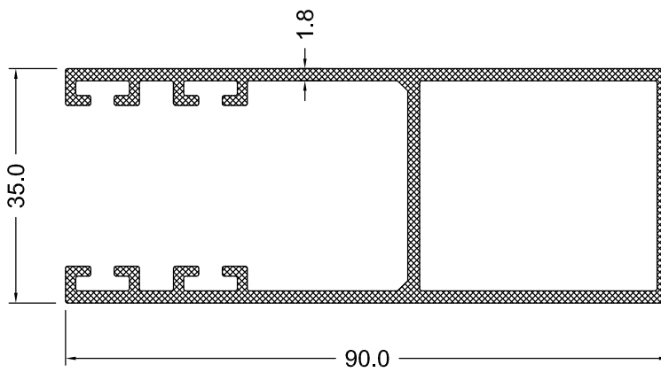
9352-18 1.379 Kg/m
