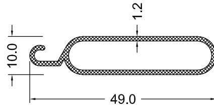
9321-12 0.334 Kg/m
