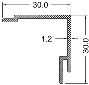
LM 52-12 0.221 Kg/m
