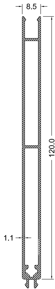
LM 11-11 0.833 Kg/m
