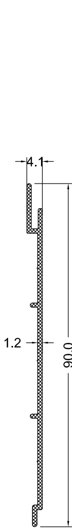
LM 1084-12 0.333 Kg/m
