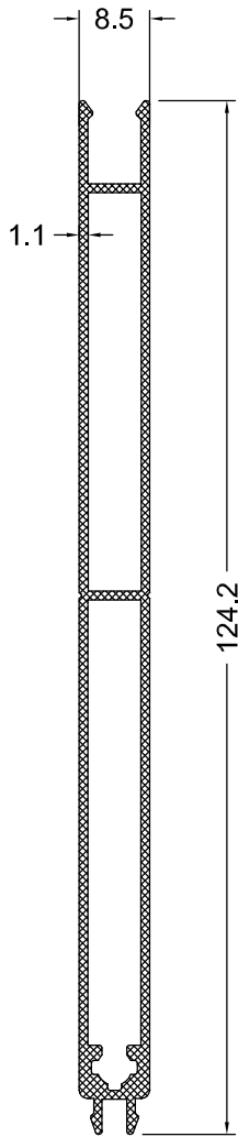
16035 0.800 Kg/m
