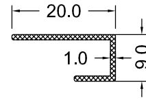
LM 53-10 0.095 Kg/m
