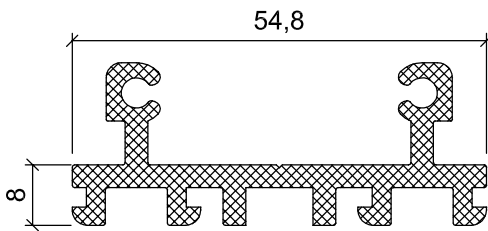
WT 71-00 0.992 Kg/m
