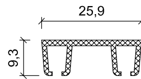
WT 55-15 0.211 Kg/m
