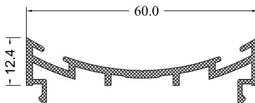
WT 57-15 0.515 Kg/m
