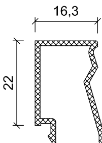
WT 46-13 0.258 Kg/m
