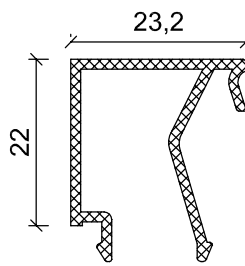
WT 44-13 0.307 Kg/m
