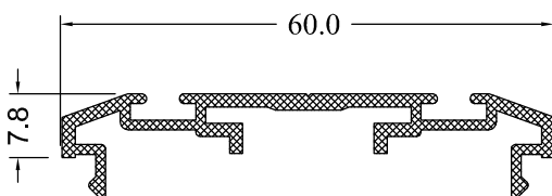
WT 56-15 0.472 Kg/m
