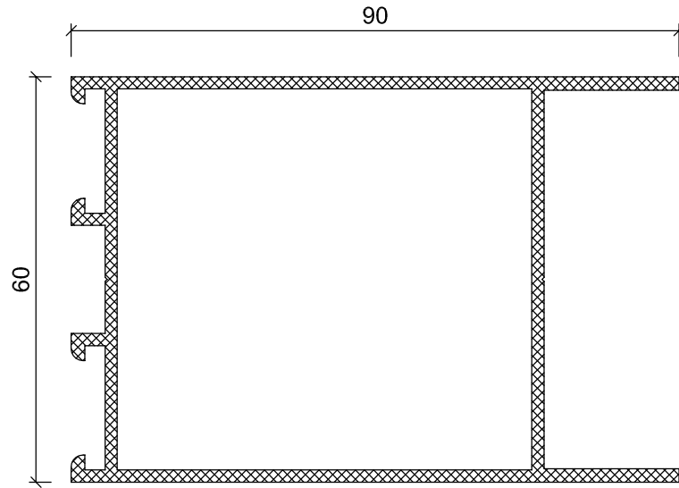
WT 21-18 1.539 Kg/m
