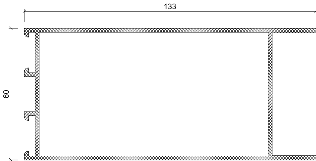
WT 22-18 1.959 Kg/m
