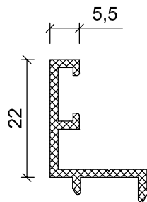
WT 47-15 0.228 Kg/m
