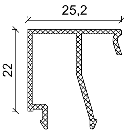
WT 43-13 0.312 Kg/m
