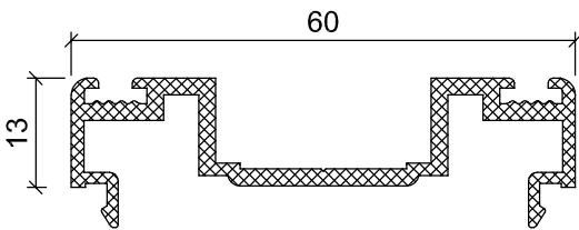
WT 52-00 0.642 Kg/m
