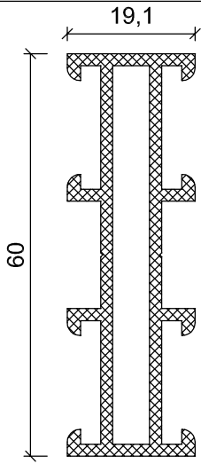
WT 10-18 0.913 Kg/m
