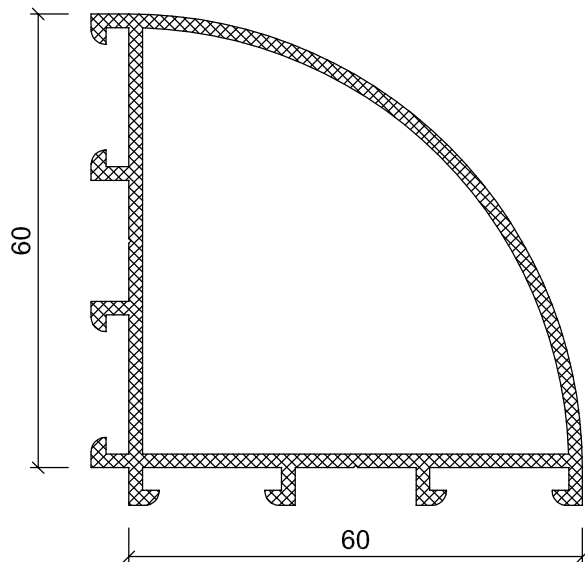
WT 62-18 1.285 Kg/m
