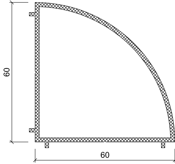
WT 61-18 1.051 Kg/m
