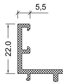
WT 48-18 0.266 Kg/m
