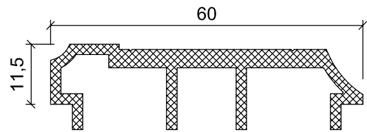
WT 53-00 0.789 Kg/m
