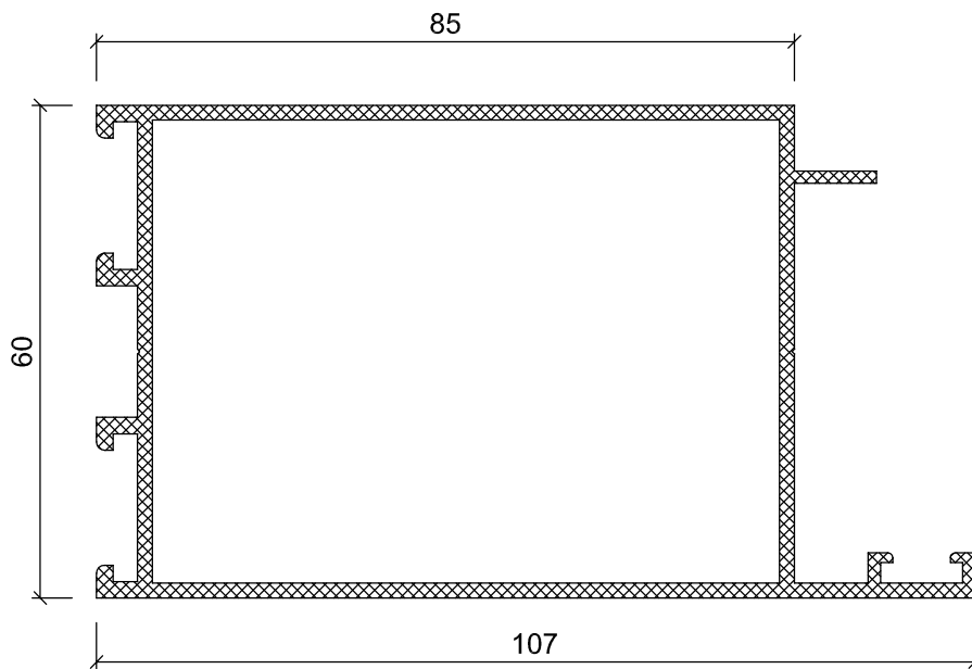
WT 32-18 1.667 Kg/m
